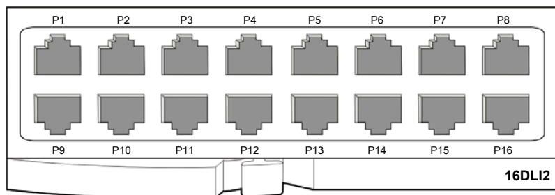
Рис. 2.14 Плата 16DLI2 - вид спереди
