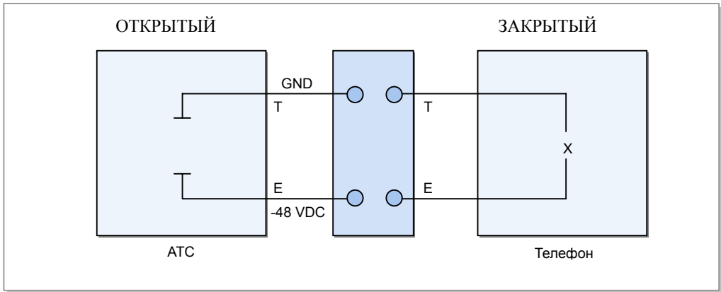
Рис. 3.1 Сигнализация аналоговых внешних линий
